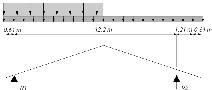
Figure 4.4 Réactions aux murs dues aux charges de gravité du Cas 3
