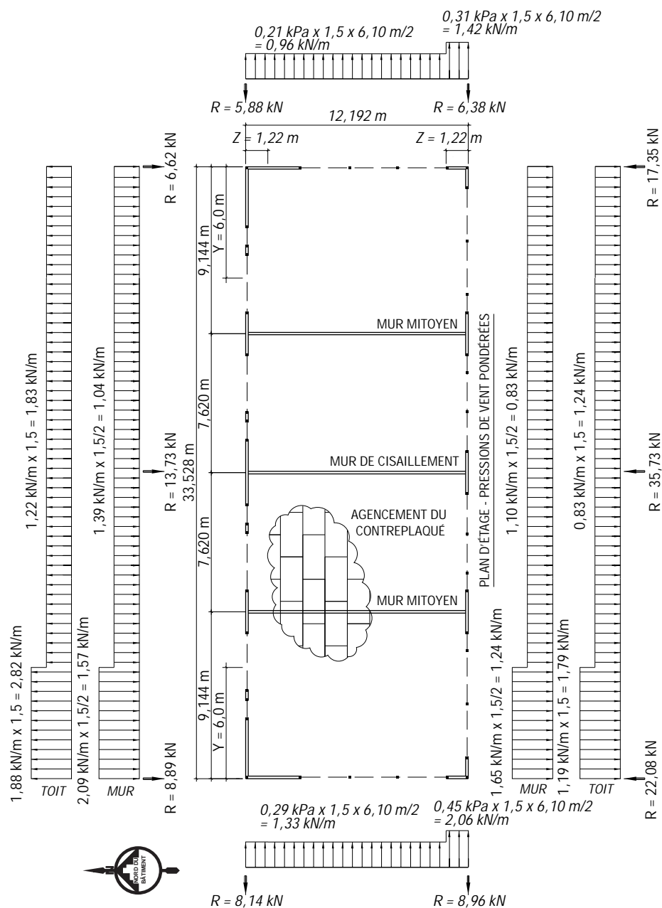
Figure 4.10 Composantes de charges latérales pondérées dues aux pressions de vent, pour le calcul des diaphragmes et des murs de cisaillement
