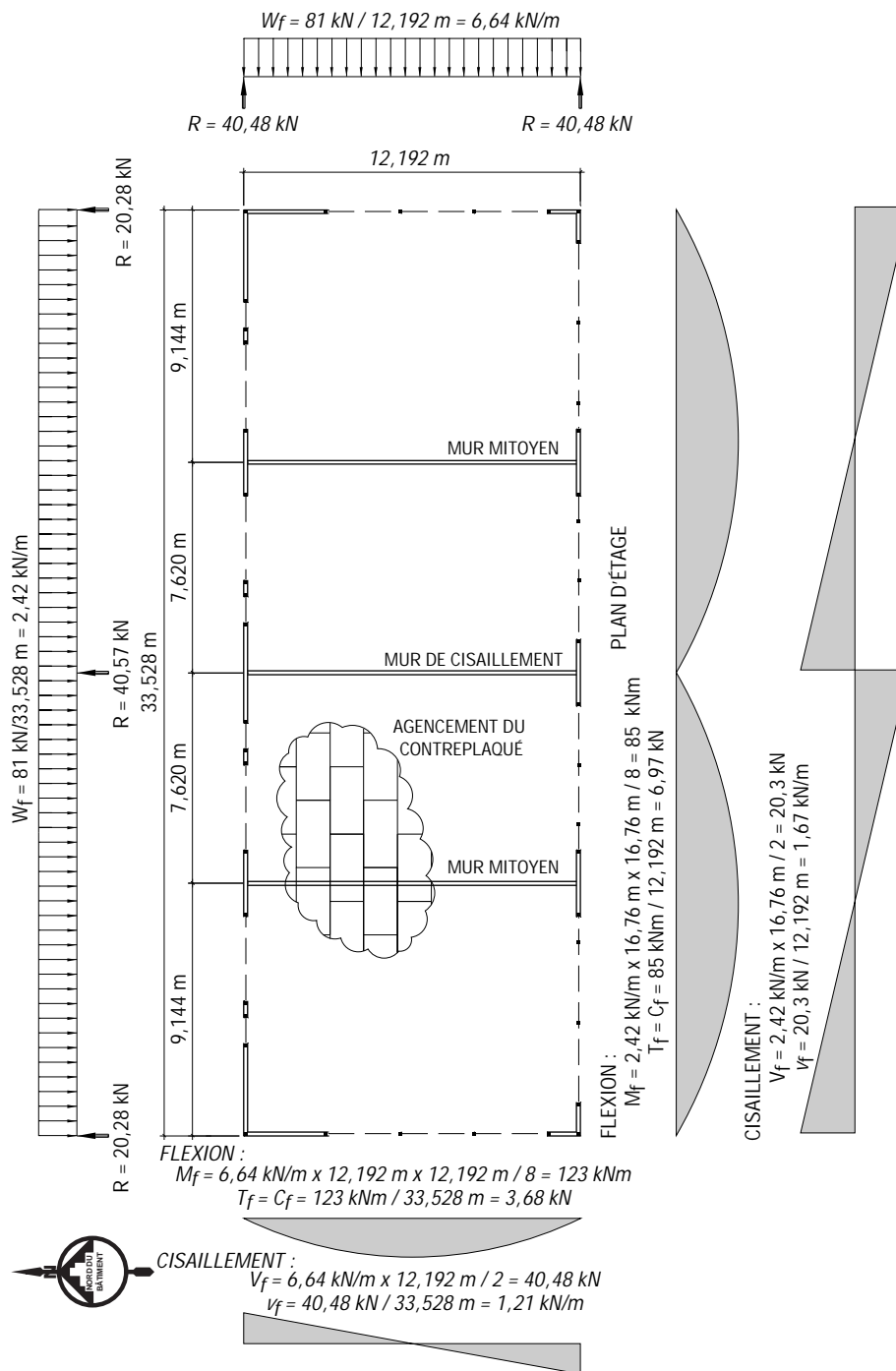
Figure 4.12 Composantes de charges latérales pondérées dues aux charges sismiques, pour le calcul des diaphragmes et des murs de cisaillement
