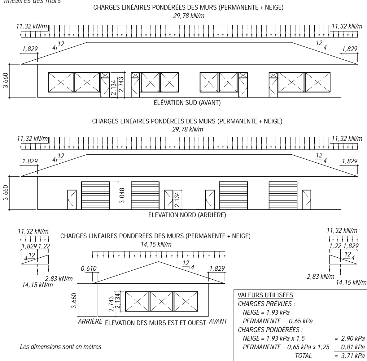
Figure 4.15 Sommaire des charges linéaires des murs
