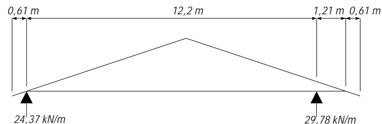
Figure 4.5 Réactions aux murs dues aux charges de gravité régissant le calcul
