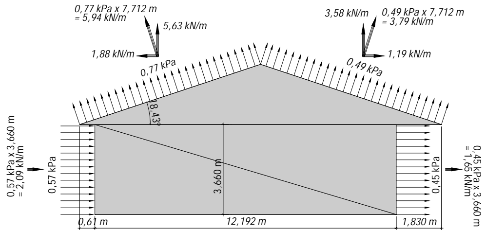
CHARGES DE VENT PRÉVUES – SECTIONS DE MUR D'EXTRÉMITÉ
